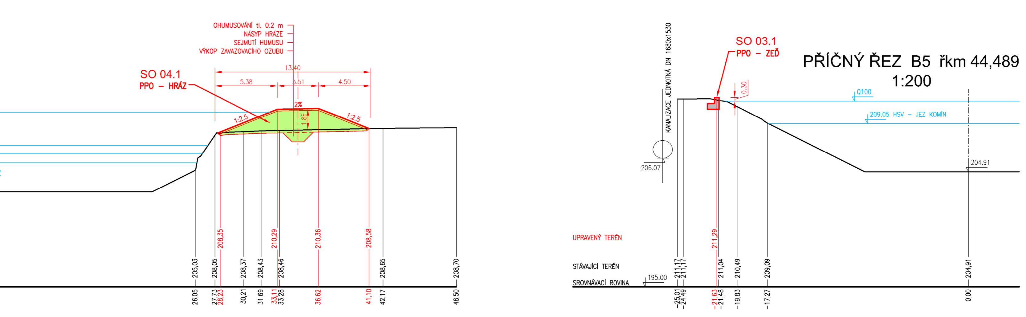
VÝŠKOVÝ SYSTÉM BpV
